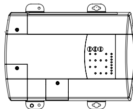
Figure 5 Orientations de montage (pont de bateau et horizontale)
