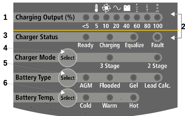
Figure 3 Panneau de commande et d'affichage d'état de bord
