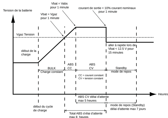
Figure 12 Cycle de charge en 2 Stage (deux phases)
