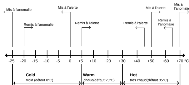
Figure 8 Seuils de température de la batterie
