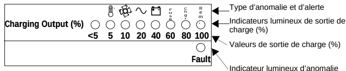
Figure 14 Indicateurs lumineux de Charging Output (%) et Fault
