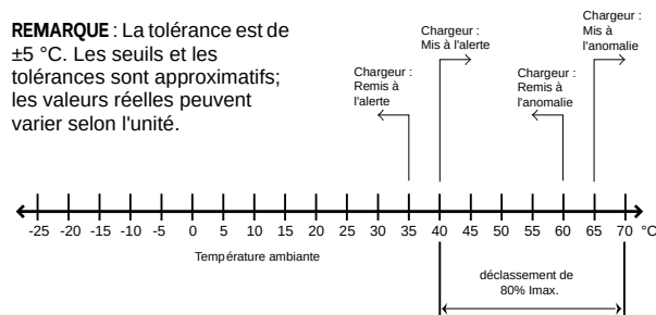
Figure 9 Seuils de température du chargeur
